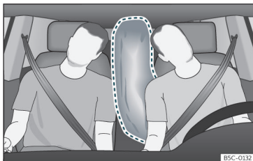
Fig. 20 Airbag centrale completamente gonfiato (area di spiegamento).
