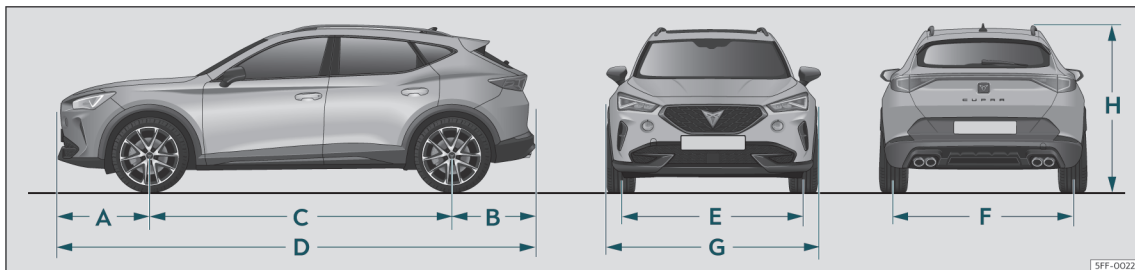
Fig. 199 Dimensioni.
